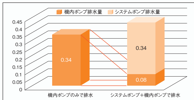
機内ポンプ排水量の比較
