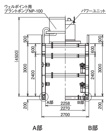
A-A矢視図
